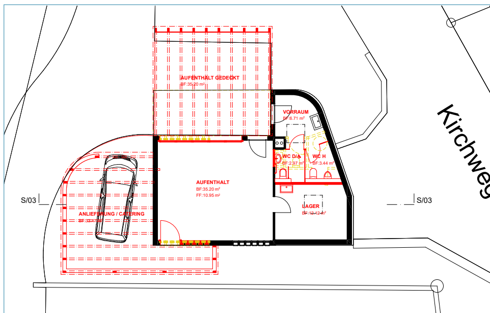
> Planansicht Erdgeschoss
