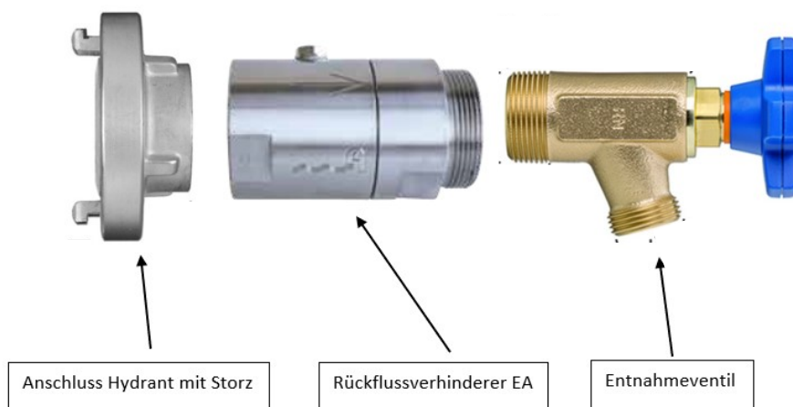
Illustration Bauwasserbezug ab Hydrant
